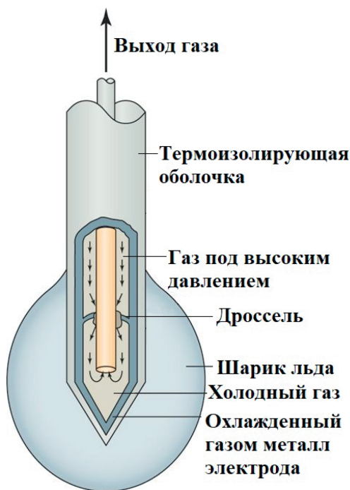
Рис. 1. Принцип работы криозонда Fig. 1. Cryoprobe operation principle
